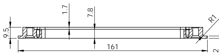
剖面 A-A 比例 1.5 : 1
