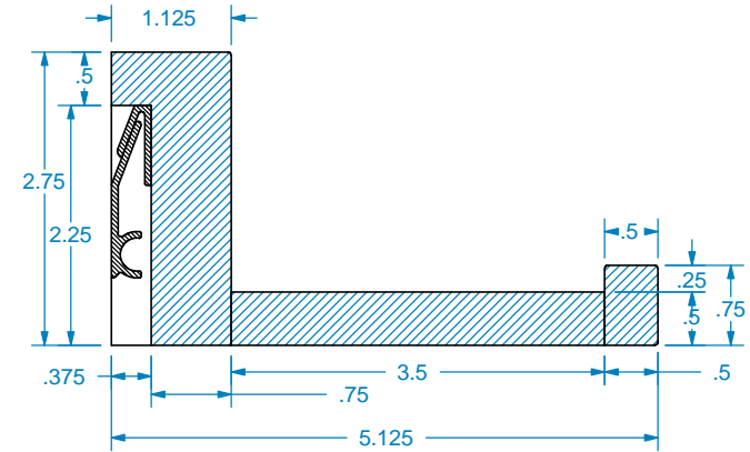
SECTION A-A SCALE 1 : 2
